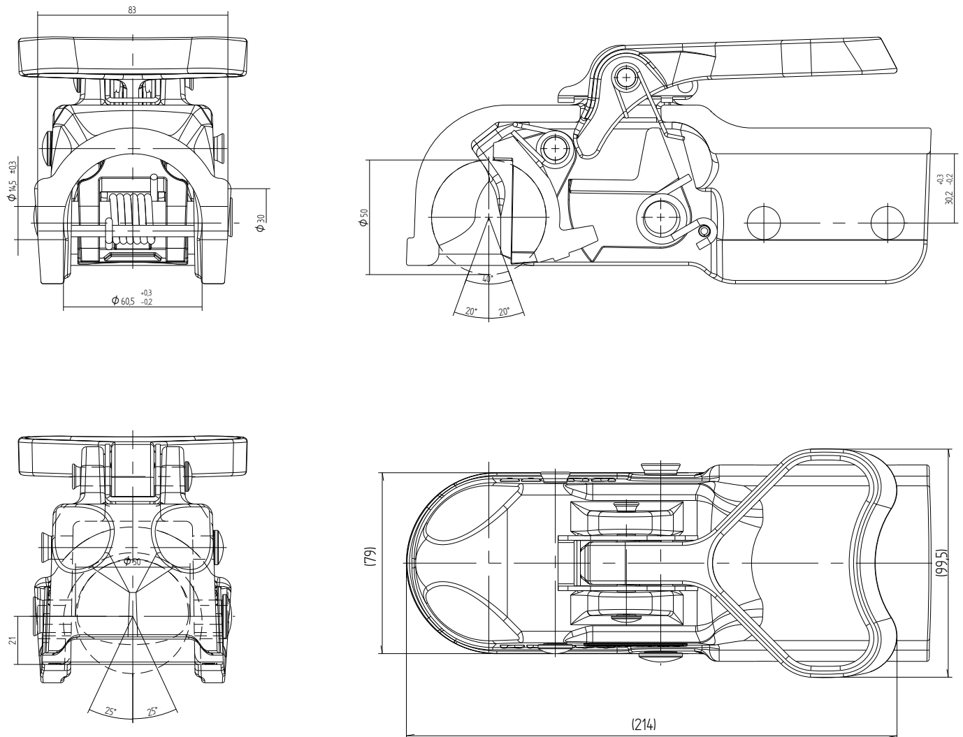
WK35-A coupling - 6E0492.001
