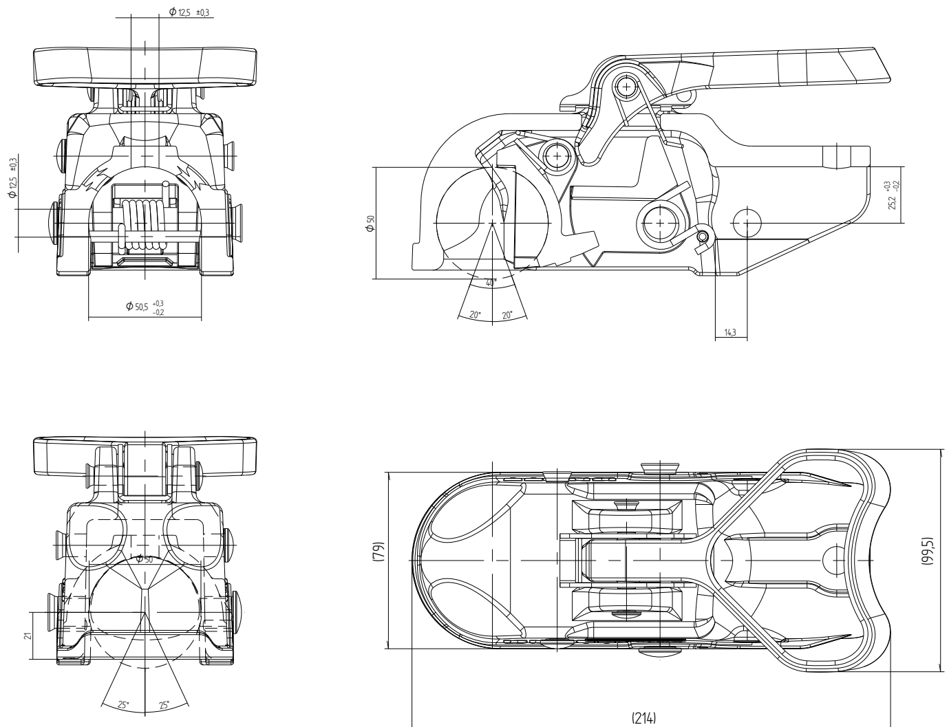
WK30-A coupling - 6E0415.001
