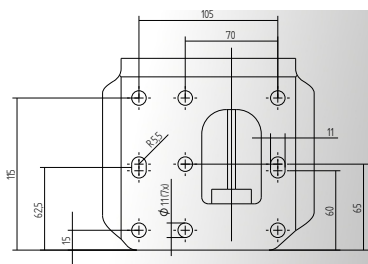
Mocowanie koła podporowego - „B”
