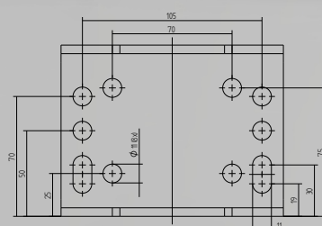
Mocowanie koła podporowego - „A”
