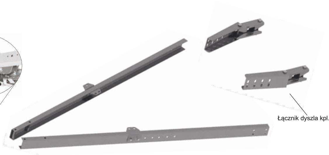
Podpora dyszla
