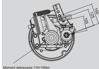
Przekrój A-A
