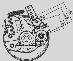
Przekrój A-A
