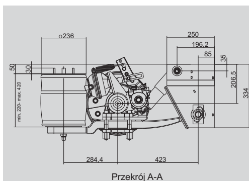
Przekrój A-A
