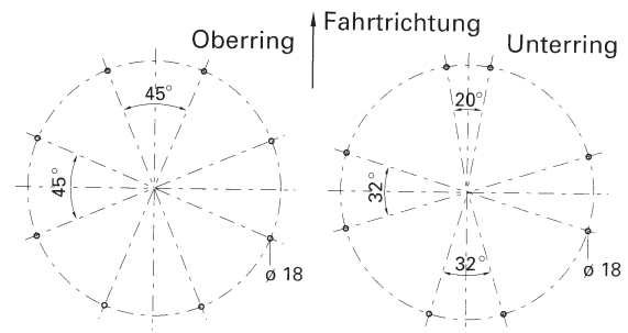
Bohrbild 1
