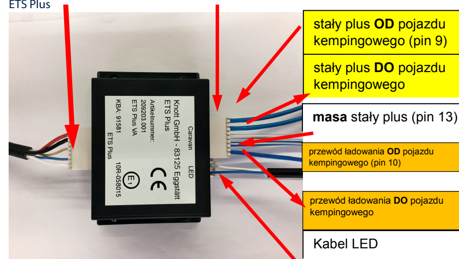
Rysunek: Okablowanie systemu ETS z układem odłączania odbiorników w pojeździe kempingowym
