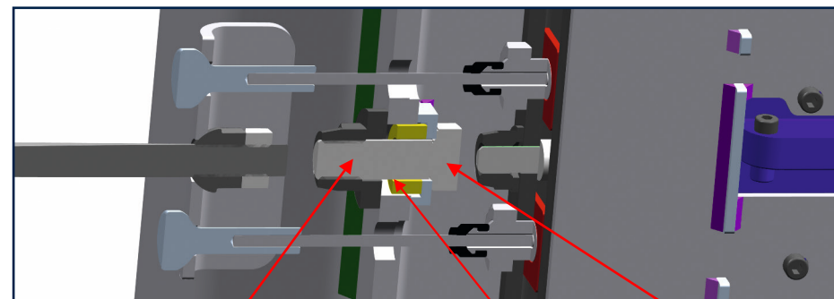
nakrętka zabezpieczająca M12 moment dokręcania 80 +10 Nm
