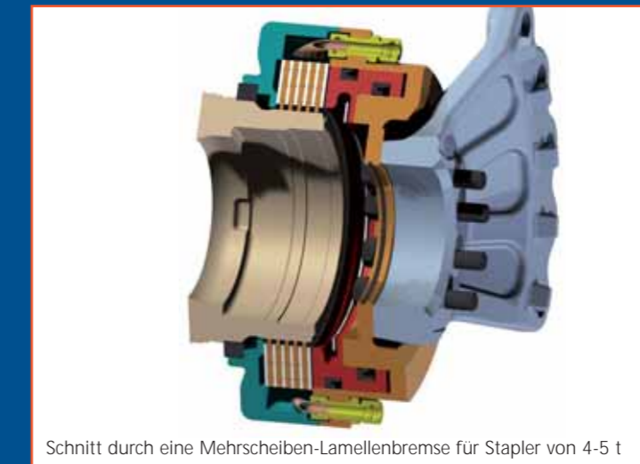
Schnitt durch eine Mehrscheiben-Lamellenbremse für Stapler von 4-5 t
